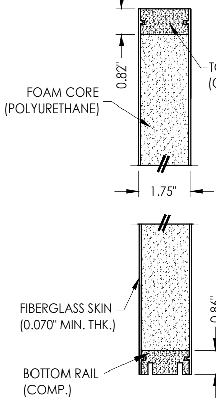
SECTION D-D
